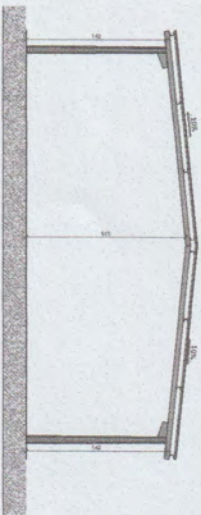
4 Corte 2 1:100
