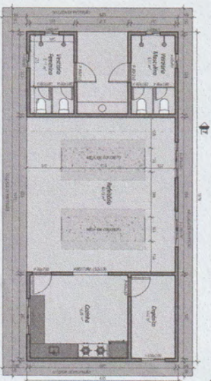
6 PLANTA BAIXA - REFEITÓRIO 1:75
